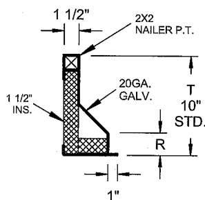
RPEJ-1 SECTION
