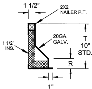
RPEJ-1 SECTION
