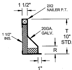
RPEJ-1 SECTION
